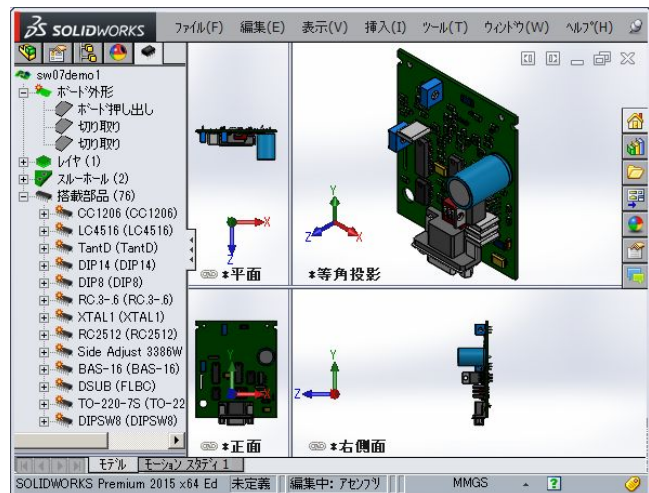
CircuitWorks で自動作成した プリント板アセンブリの詳細モデル
